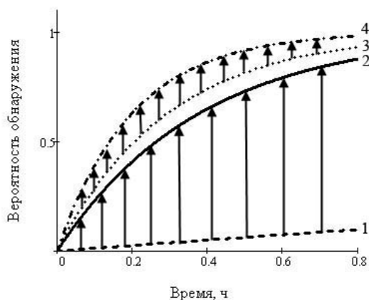
Рис. 7. Вероятности обнаружения корабля (1), корабля вместе с кильватерным следом (2) в условиях активных маскирующих помех и корабля (3), корабля вместе с кильватерным следом (4) одиночным разведчиком
