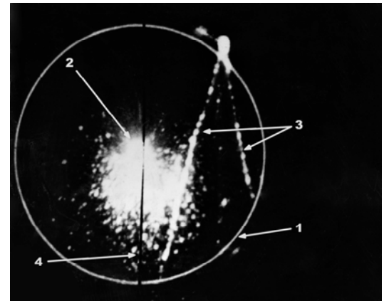
Рис. 2. Радиолокационное изображение расходящихся корабельных волн:
